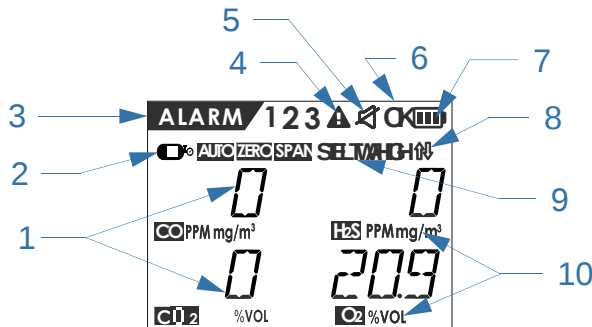
Рисунок 4 - Дисплей первого типа
