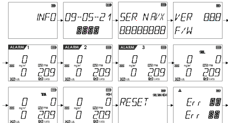
Рисунок 11 – Последовательность отображения информации на дисплее при включении и выключении прибора
