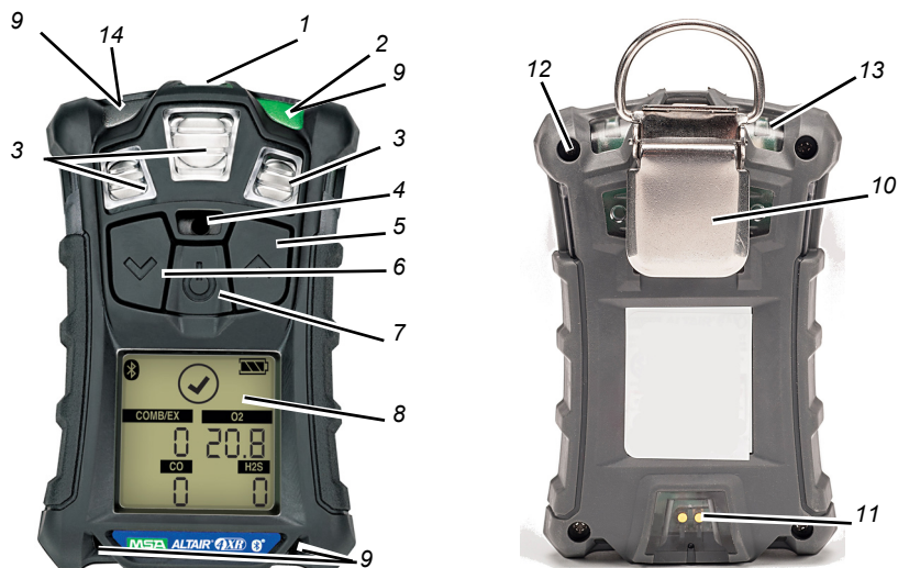
Рис. 1 Обзор устройства
