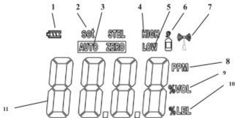
Рис.2 Дисплей газоанализатора ГАНК-П2
